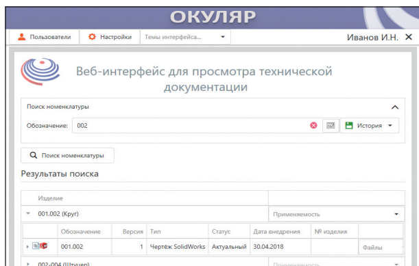
Рис. 2. Веб-интерфейс
